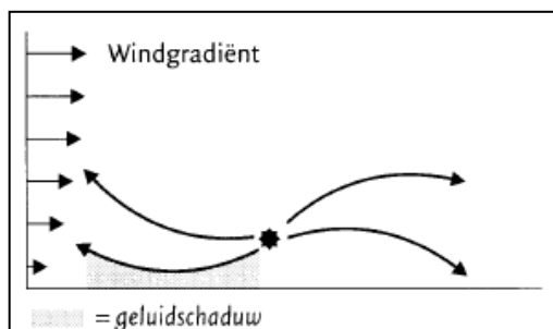
Figuur 1: windgradiënt
