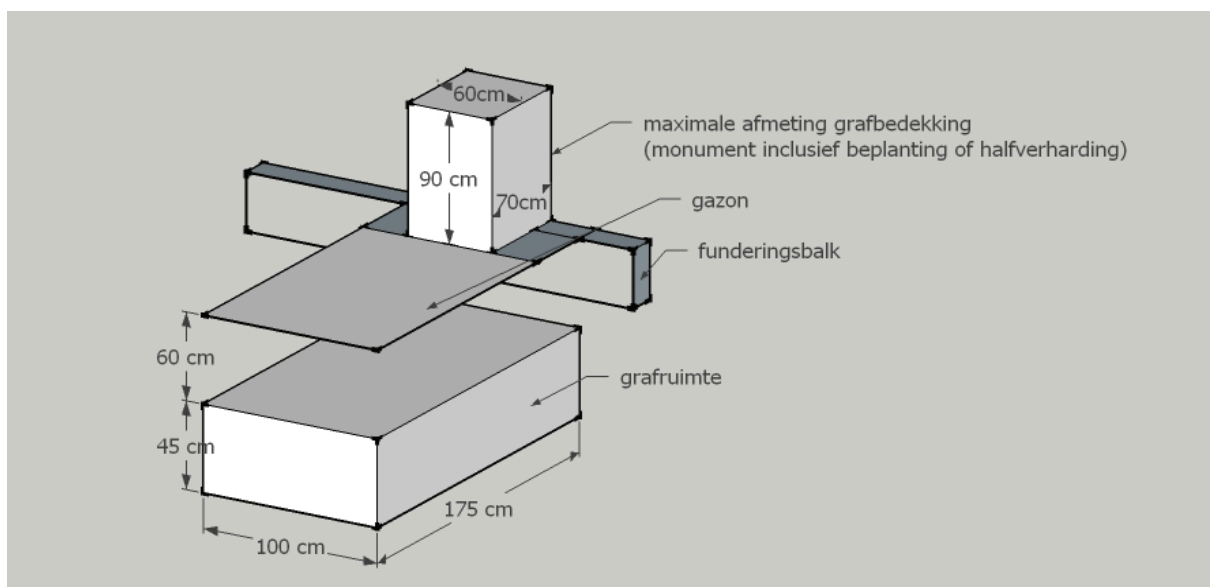
Afbeelding 2: afmetingen bij een kindergraf
