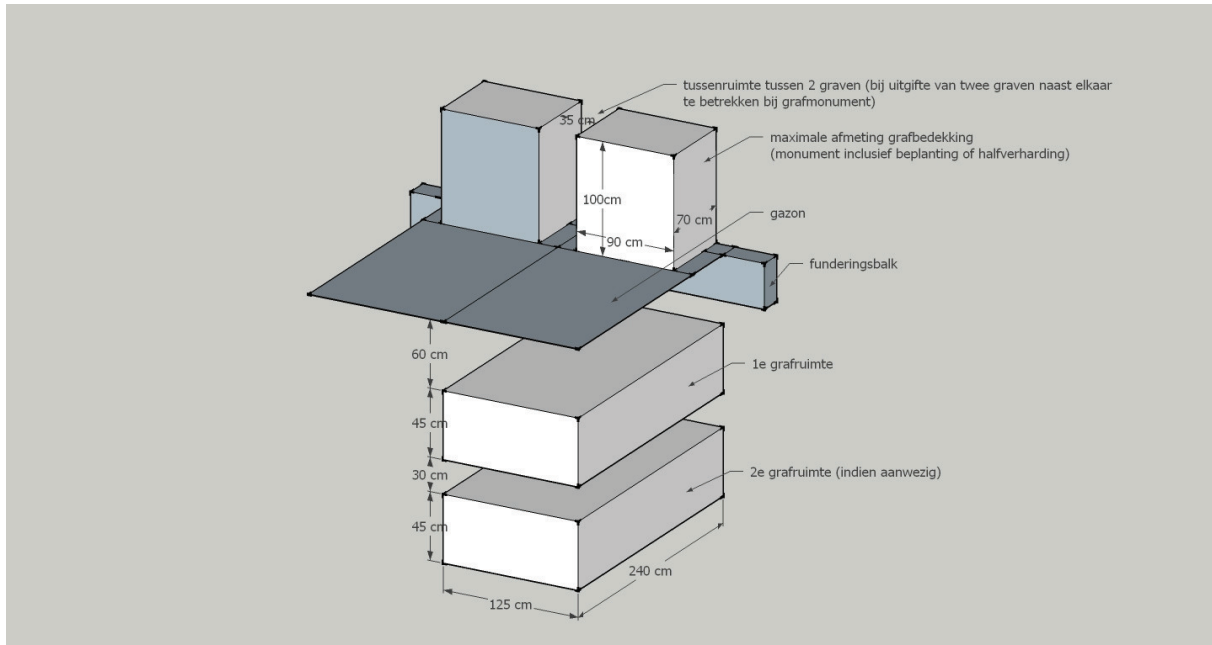
Afbeelding 1: afmetingen bij een particulier en algemeen graf
