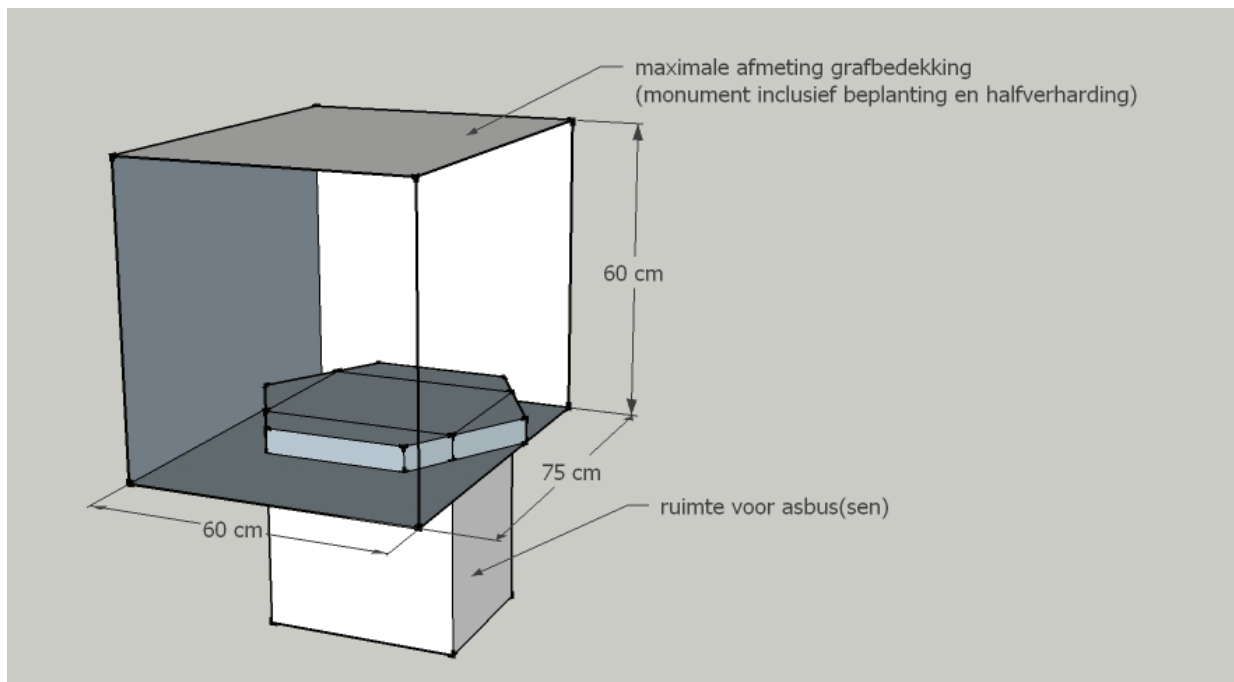
Afbeelding 3: afmetingen bij een urnengraf
