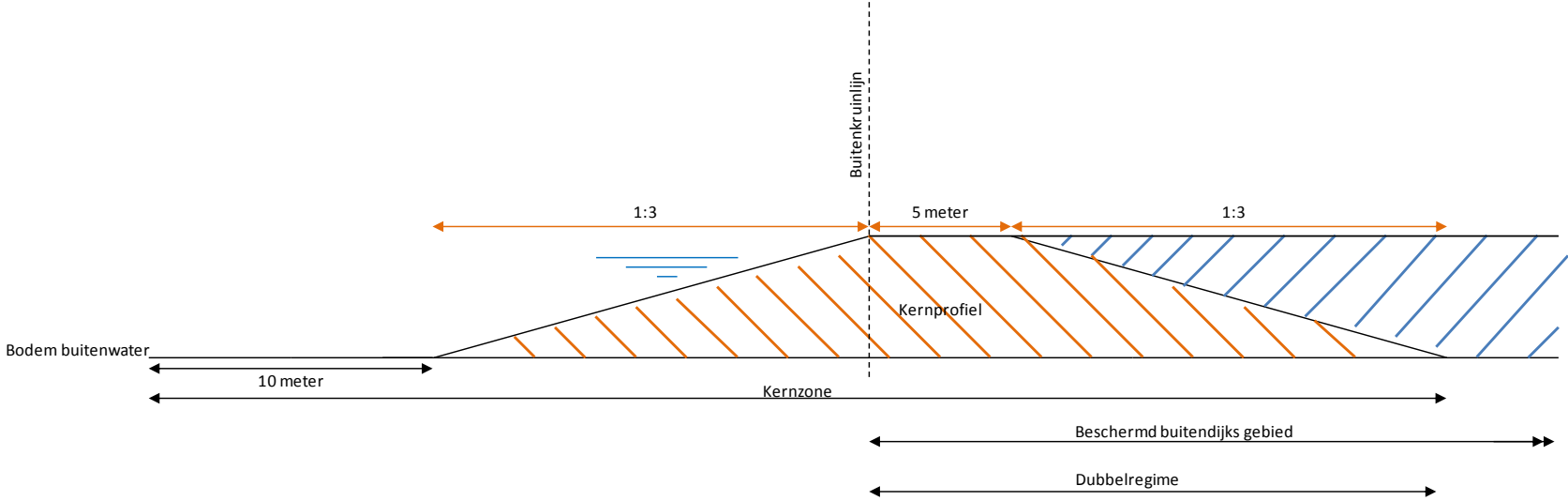
Figuur Zonering traditionele waterkering
