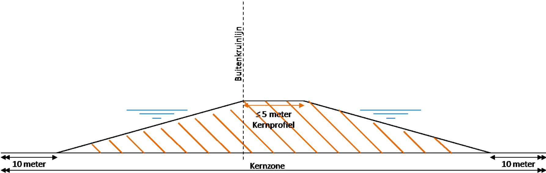
Figuur Strekdam tbv bescherming regionale waterkering kruin < 5 meter
