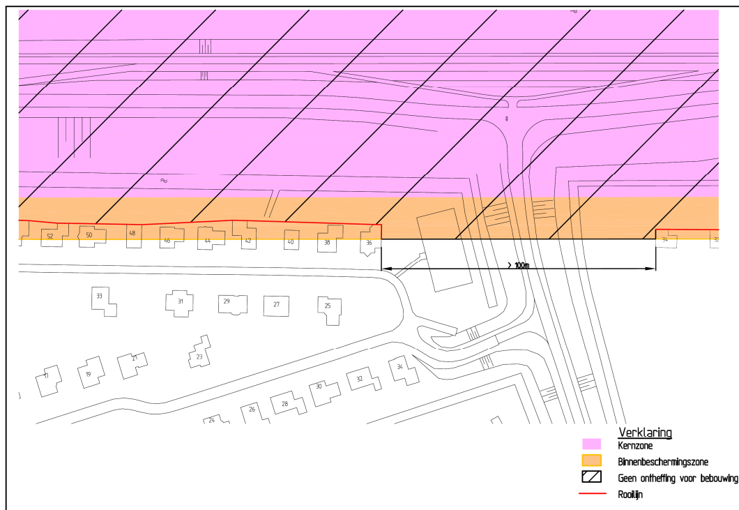
Figuur 3 Toelichtende tekening bij beleidsregels bouwactiviteiten (in de gearceerde zones zijn enkele bouwactiviteiten zoals beschreven in dit hoofdstuk onder voorwaarden mogelijk)
